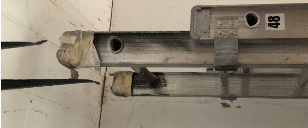
Fotografía 5. Parte superior de la escalera de extensión con marcas de quemaduras en donde la escalera tocó al cable de electricidad.
